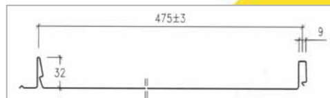
Tagpladens modulbredde og højde
